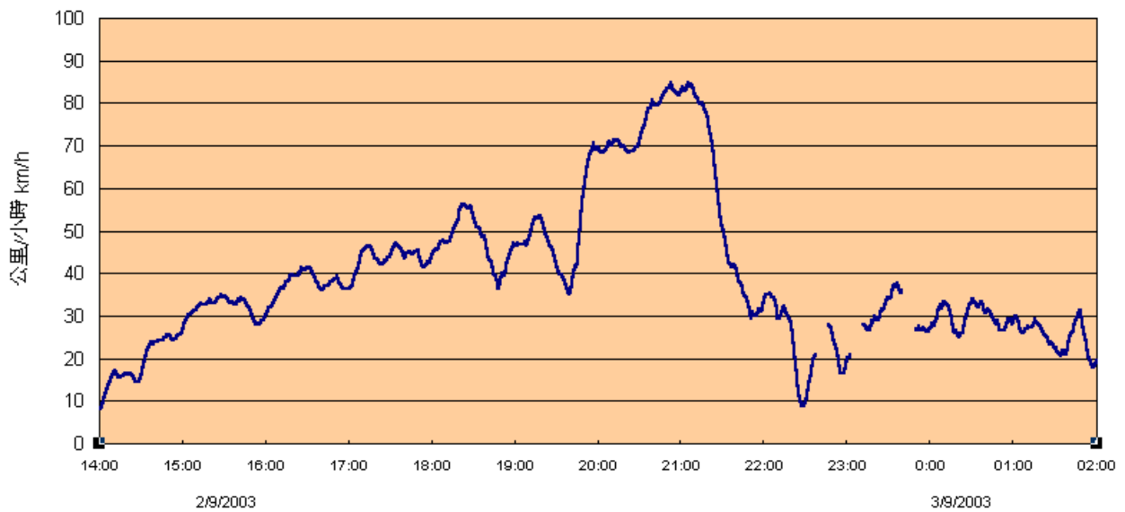
圖 3.4.3.b 九龍天星碼頭錄得的十分鐘平均風速的變化情形。
