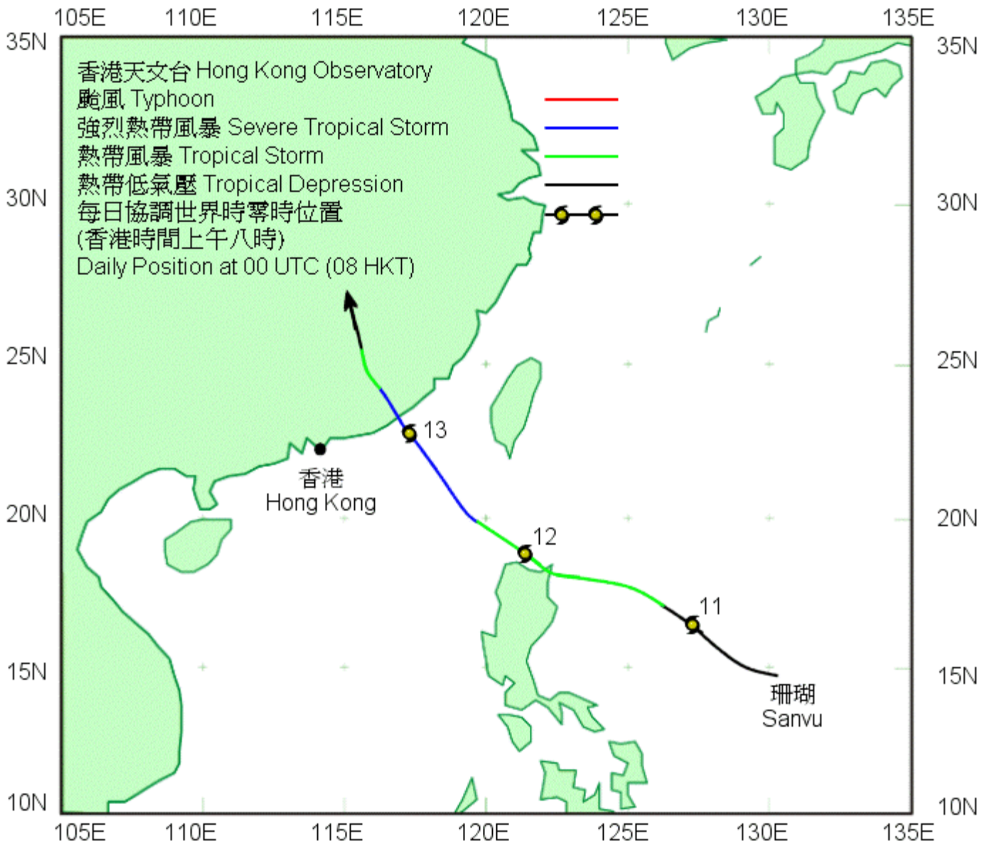
圖 3.1.1 二零零五年八月十日及十四日珊瑚 (0510) 的路徑圖 Figure 3.1.1 Track of Sanvu (0510) on 10 - 14 August 2005.
