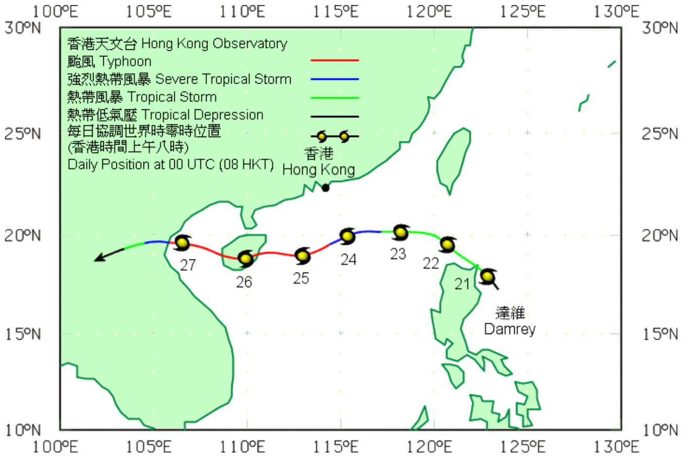
圖 3.3.1 二零零五年九月二十一日至二十八日達維 (0518) 的路徑圖。 Figure 3.3.1 Track of Damrey (0518) on 21 - 28 September 2005.
