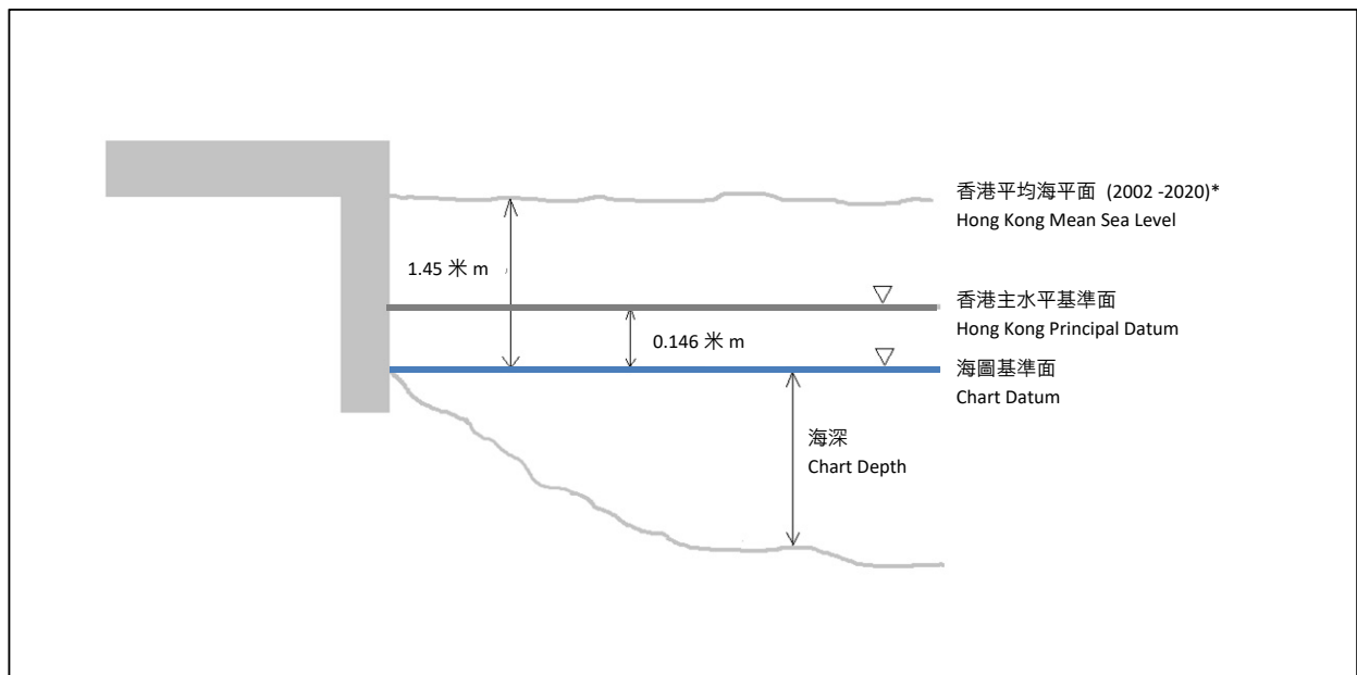
香港高程基準示意圖
