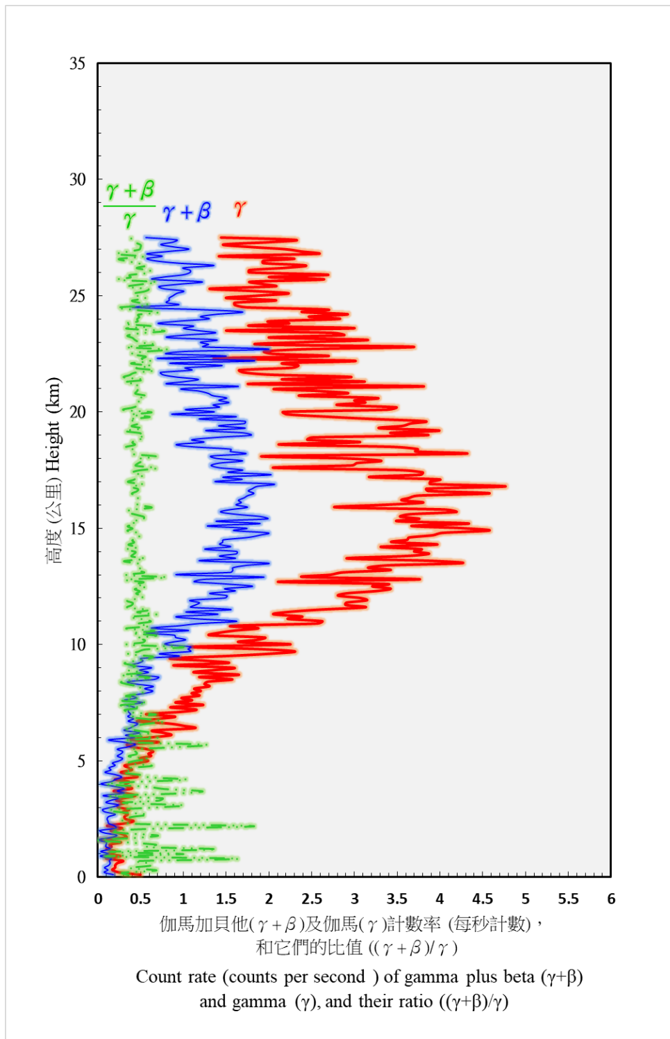
圖 7. 二零二二年在京士柏進行的高空輻射探測之平均大氣放射性垂直廓線 (探測日期為：六月十三日及九月二十六日)。
