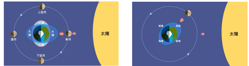
潮汐的示意圖 (不依比例)
